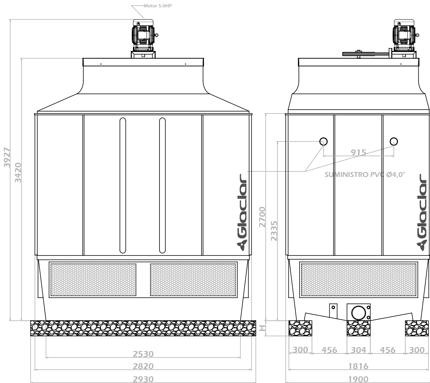
VISTA LATERAL
