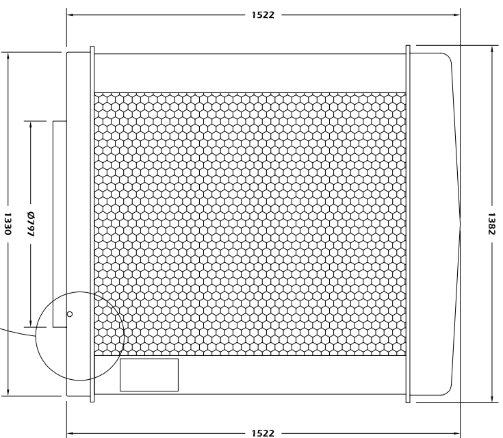
VISTA POSTERIOR
