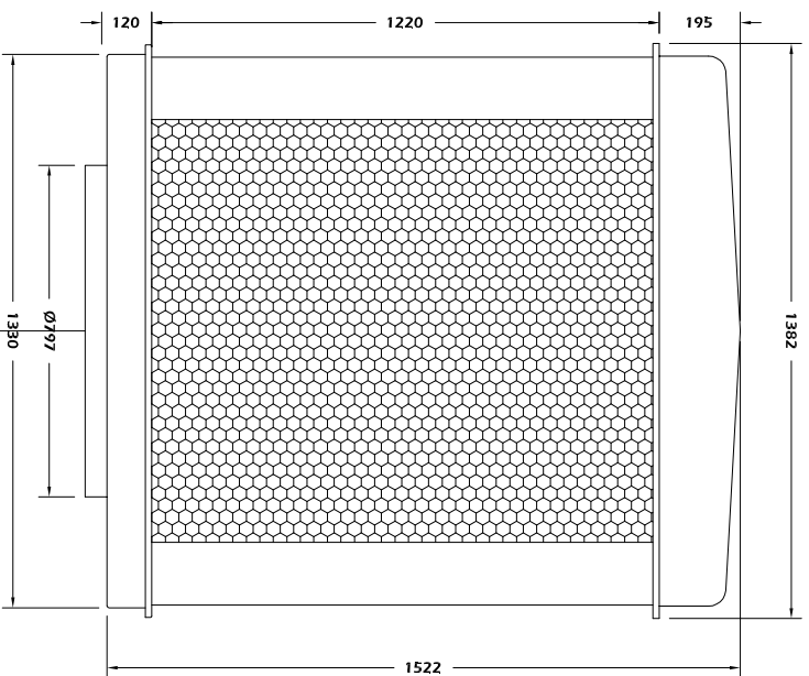
VISTA LATERAL
