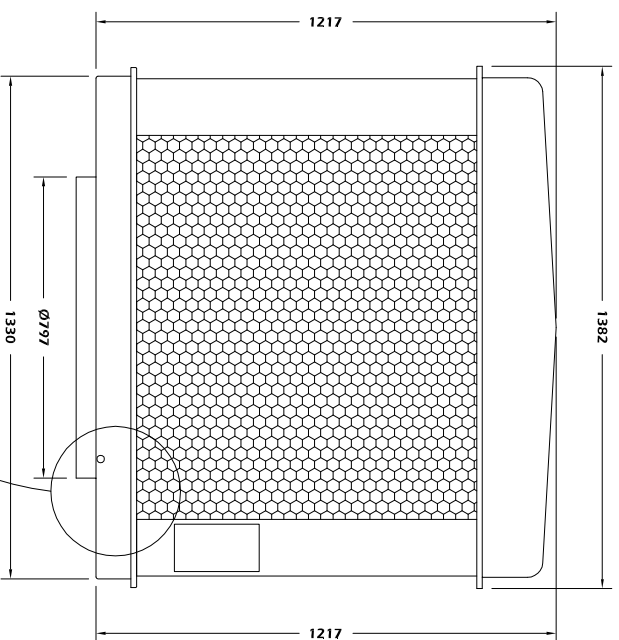
VISTA POSTERIOR
