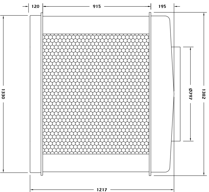
VISTA LATERAL
